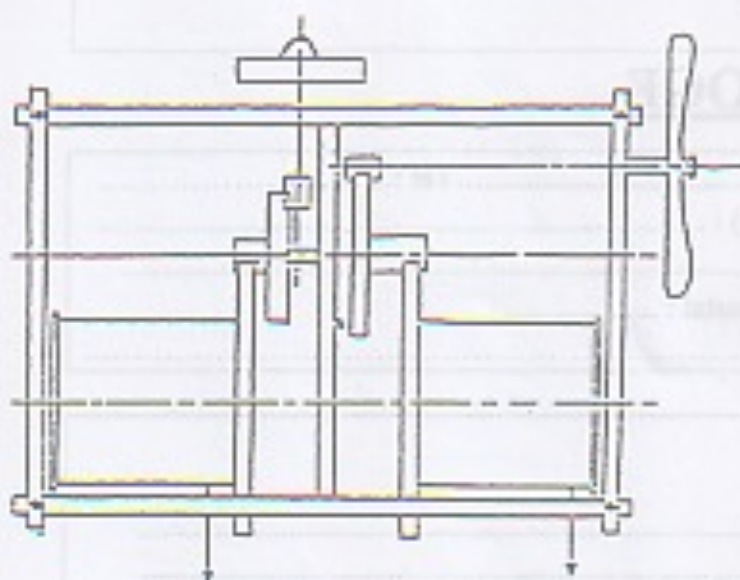
Horloge d'édifice verticale à rouages l'un derrière l'autre
