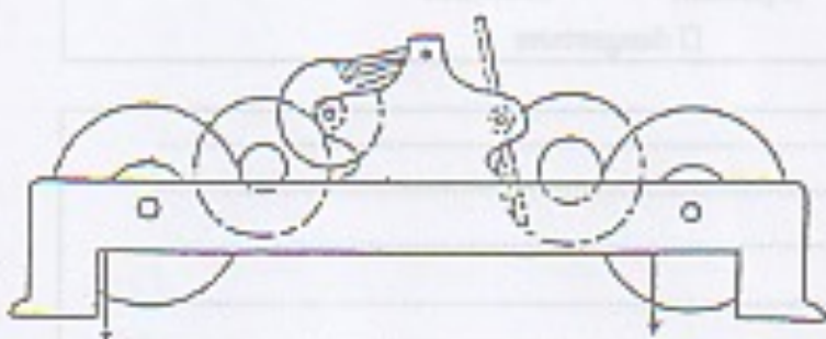
Horloge d'édifice à rouages horizontaux
